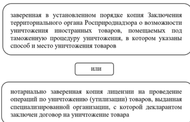
Рис. 8 Перечень документов
